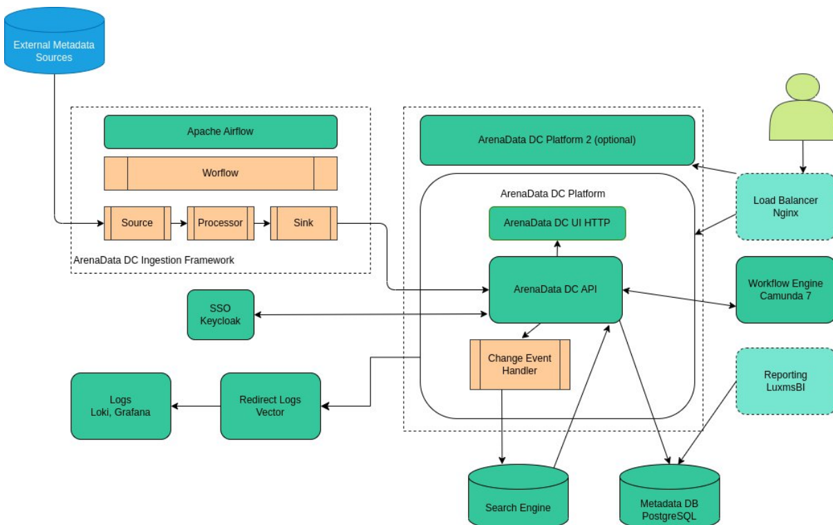
Рисунок 1 Высокоуровневая архитектура платформы Arenadata Catalog
