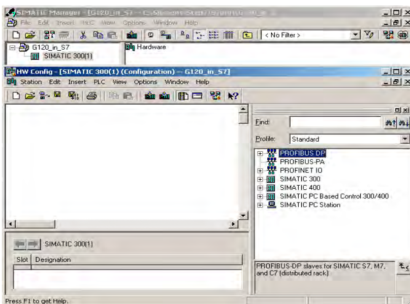
Изображение 5-25 Открыть аппаратную конфигурацию
