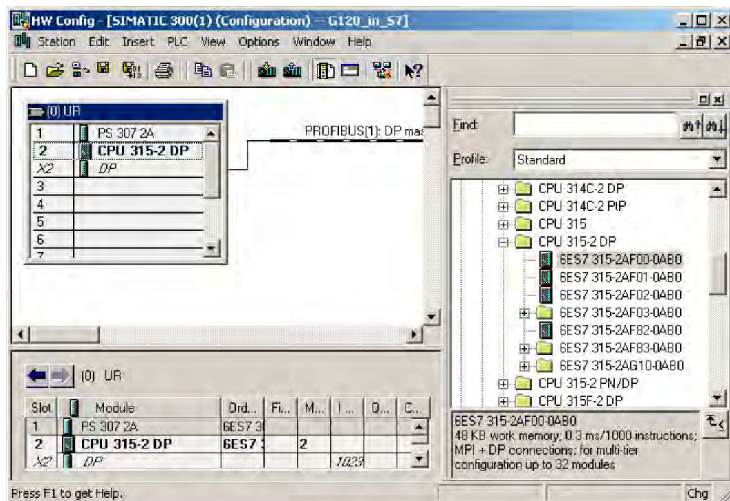
Изображение 5-26 Вставить станцию SIMATIC 300 с сетью PROFIBUS DP
