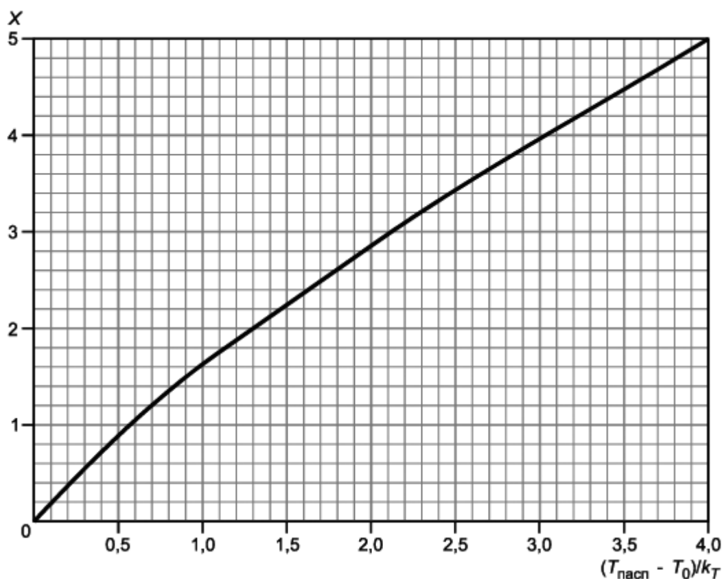
Рисунок В.2 - График для интерполяционного определения времени активации спринклерного
