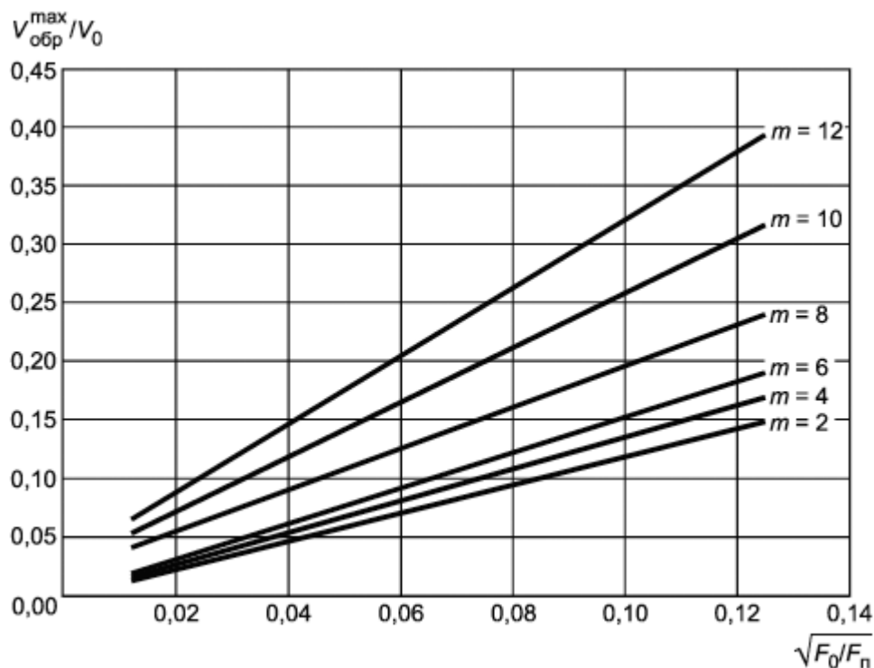
Рисунок Ж.2 - Зависимость максимальной скорости в обратном потоке от параметра
