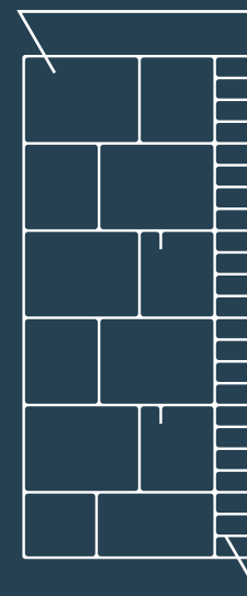
кирпичная кладка из облицовочного кирпича — 120 мм
