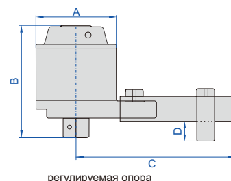
регулируемая опора
