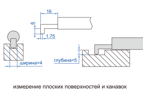
датчик глубоких канавок (опция), код ISR-C200-SB121
