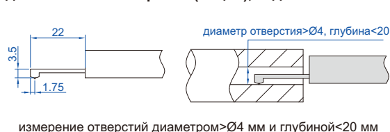
датчик малых отверстий (опция), код ISR-C200-SB31
