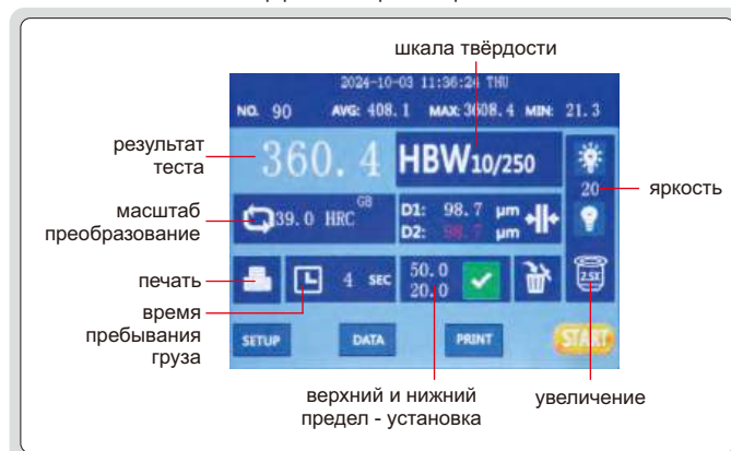
интерфейс измерения Бринелля
