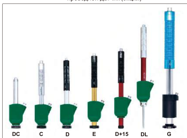
проводной датчик (опция)
