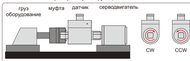
пример контроля крутящего момента
