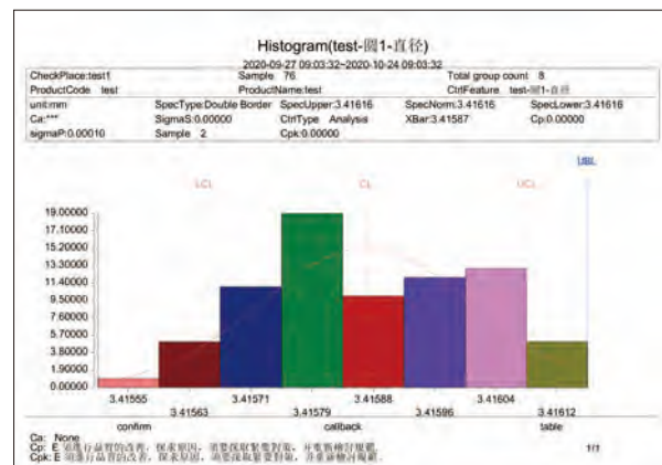
гистограмма
