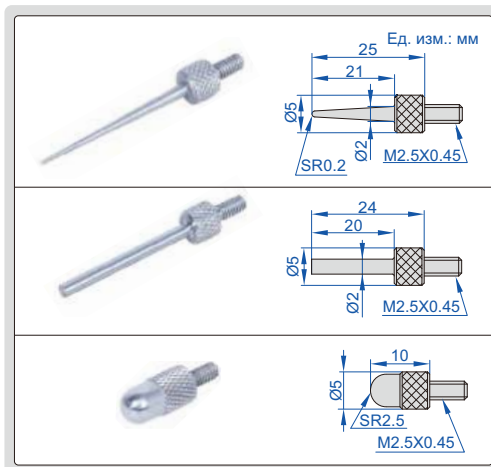
измерительные наконечники (в комплекте)
