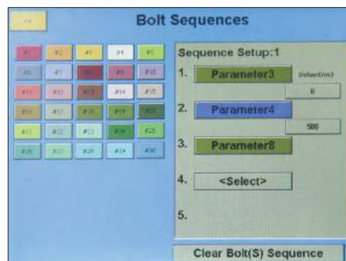
интерфейс параметров согласования винтовой последовательности
