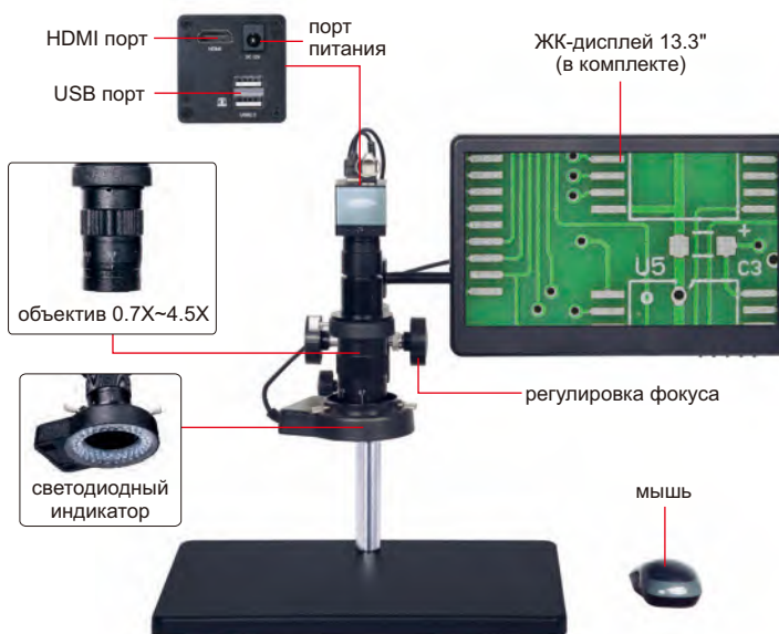
5318-MD60 (без подставки)
