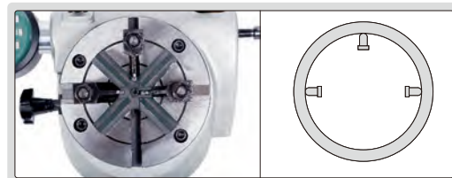
зонд для пазов для измерения внутреннего диаметра
