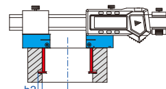
измерение внутреннего диаметра паза с помощью сферической измерительной поверхности (глубина h2 \leq 7.5 мм)
