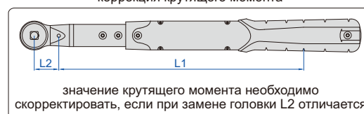
коррекция крутящего момента
