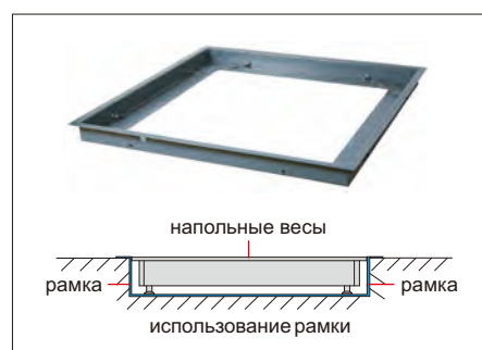
рама (опция)
