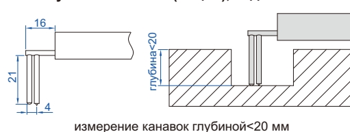
датчик глубоких канавок (опция), код ISR-C200-SB121
