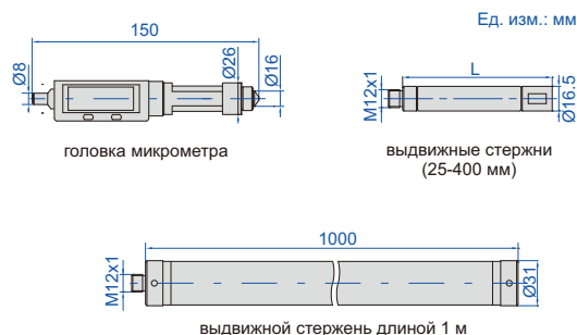
выдвижной стержень длиной 1 м
