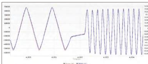
режим управления триггером, переключение формы сигнала управления
