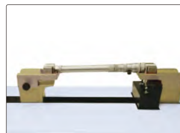
установка нуля и калибровка трубчатых внутренних микрометров
