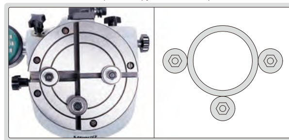
измерение наружного диаметра
