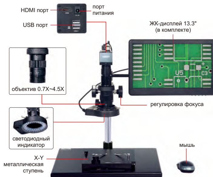
5318-MD60-XY (с подставкой)
