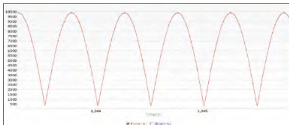
полусинусоидальная волна
