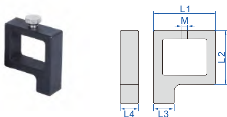
Упорный блок (опция)
