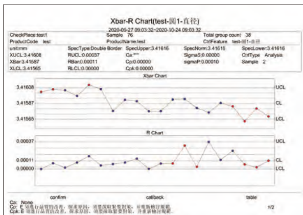
диаграмма Xbar-R
