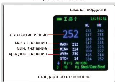
отображение статистики
