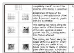
шаг 3: определение степени адгезии по осыпанию
