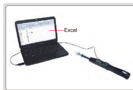
кабель передачи данных (опция), вывод сигнала клавиатуры через кабель передачи данных
