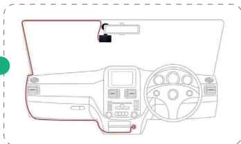
Способ прокладки кабеля В:
