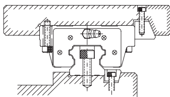
С помощью регулировочного клина
