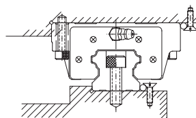
С помощью игольчатого ролика
