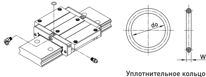
Уплотнительное кольцо
