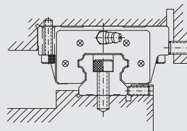
С помощью прижимного винта
