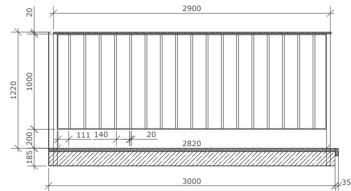
Вид сбоку
