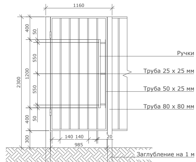
Калитка
