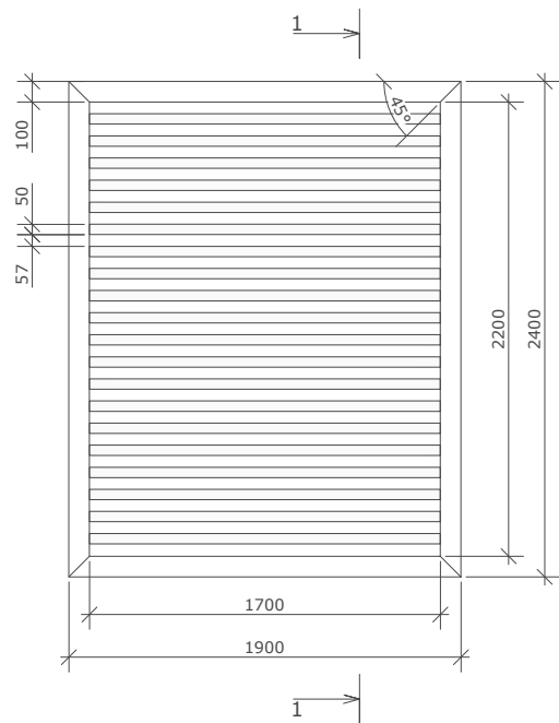
Вид спереди
