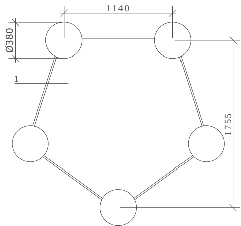
Вид сверху
