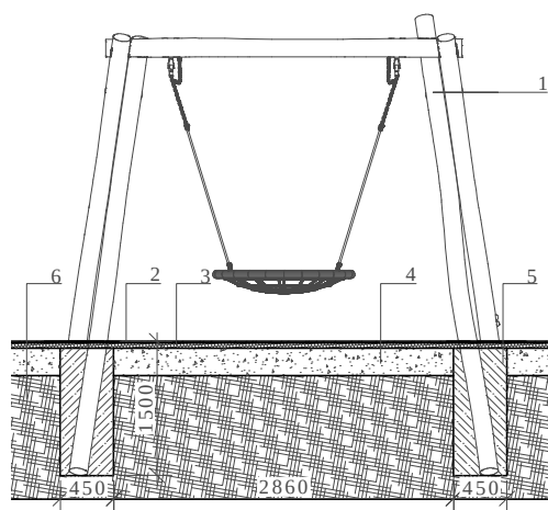
Вид спереди
