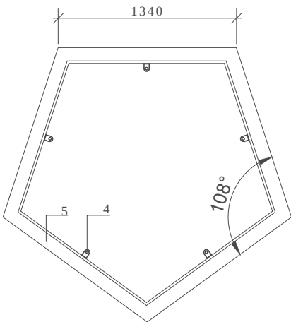
Габаритные размеры основания
