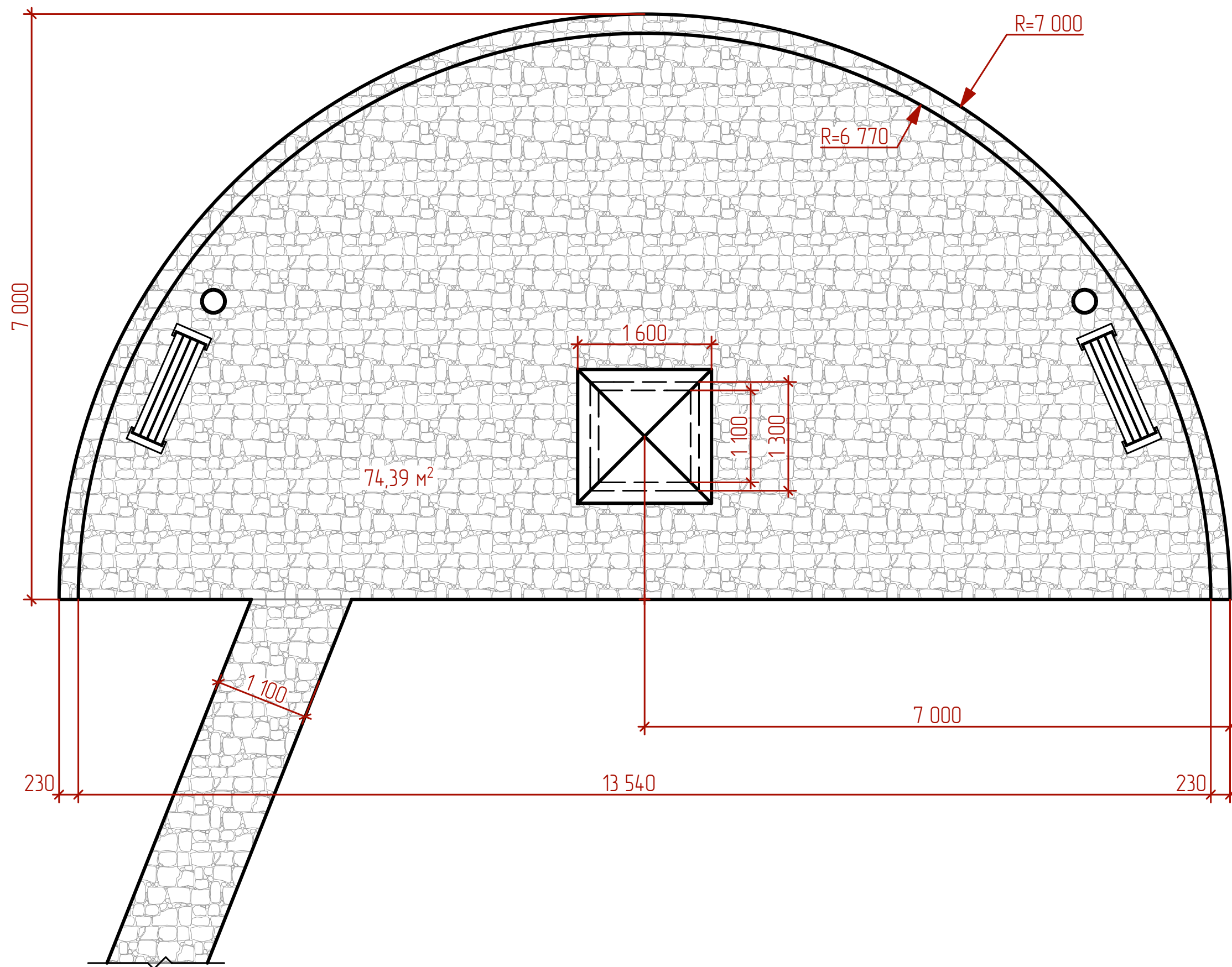
Схема площадки с часовней М 1:50
