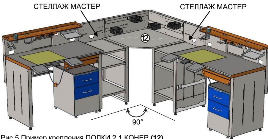
Рис.5 Пример крепления ПОЛКИ 2.1 КОНЕР (12) к столам и СТЕЛЛАЖ МАСТЕР, левое и правое исполнение
