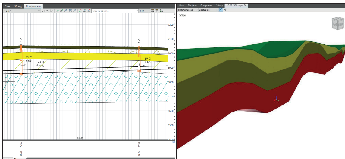
Геологическая модель местности
