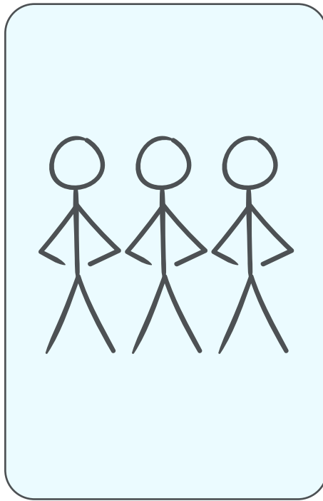
Вода
