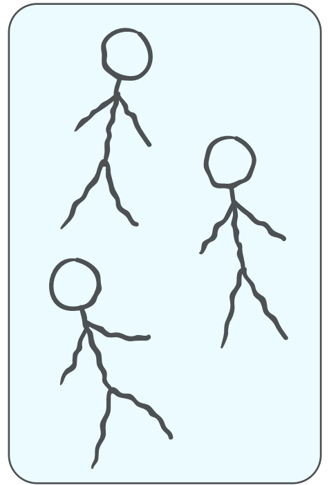
Пар
