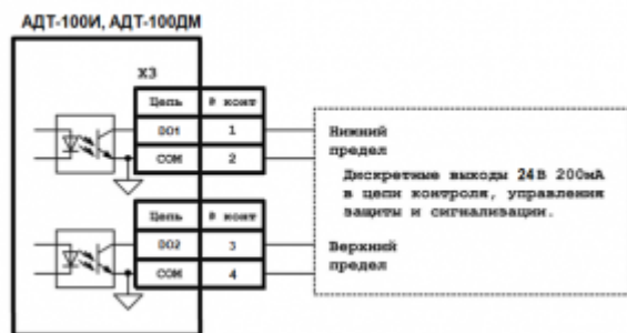
Рисунок А.7 – Схема подключения цепей дискретных выходов
