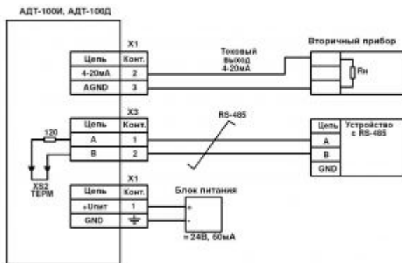
Рисунок А.3 – Схема подключения RS-485
