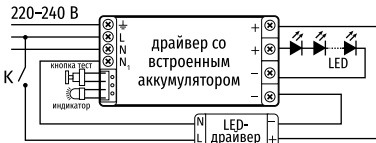
Схема подключения БАП в светильнике ДВО-15-А
