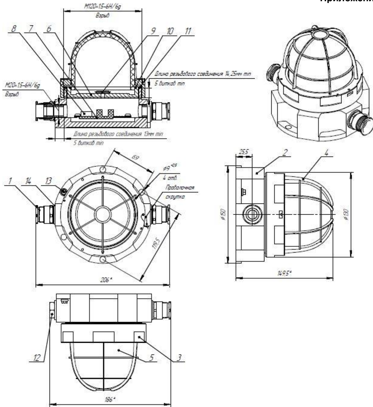
Рис. А1 Конструкция светового оповещателя ОРБИТА МК М2 - С
