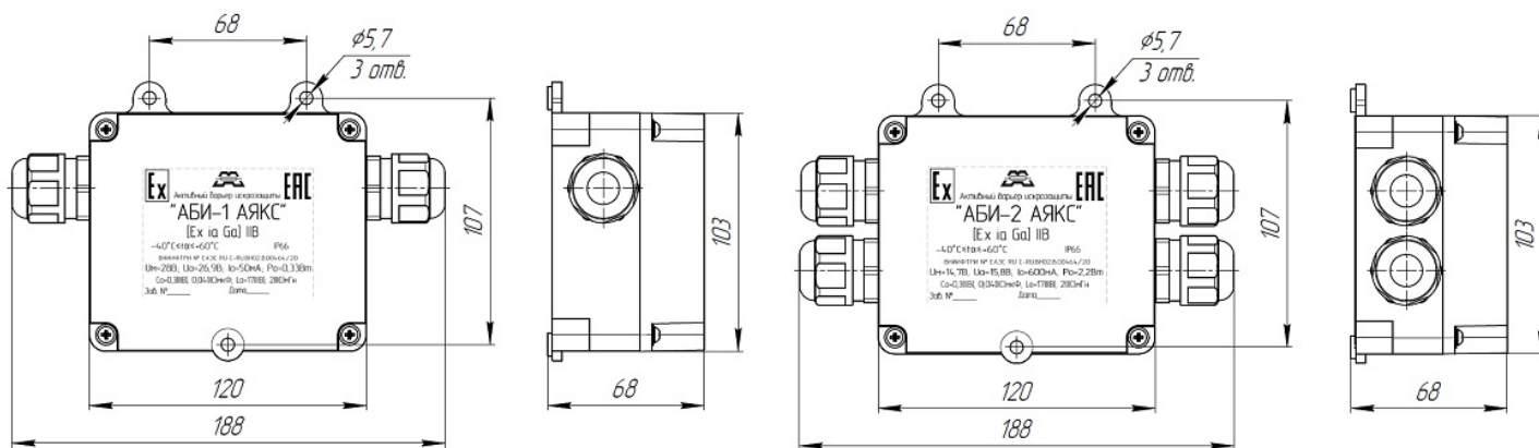
Рис.2 – Установочные размеры АБИ-1 АЯКС, АБИ-2 АЯКС
