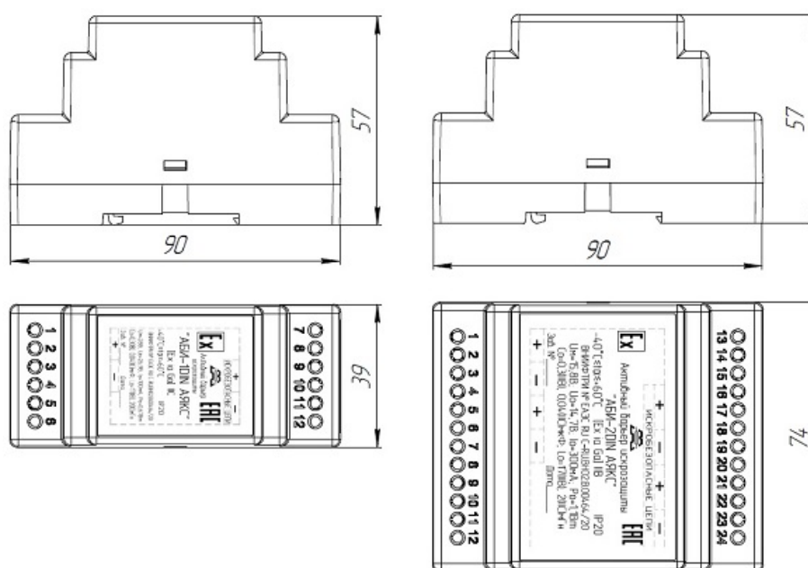
Рис.1 – Установочные размеры АБИ АЯКС на DIN рейку.
