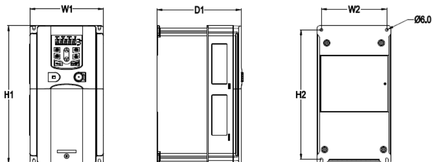
Рисунок В-3 Настенный монтаж для моделей 0R7G-15G/018P
