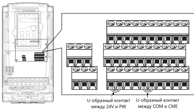
Рис. 4-21. U-образный контакт
