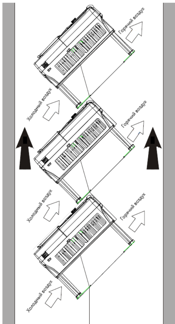
Рис. 4-6 Наклонная установка
