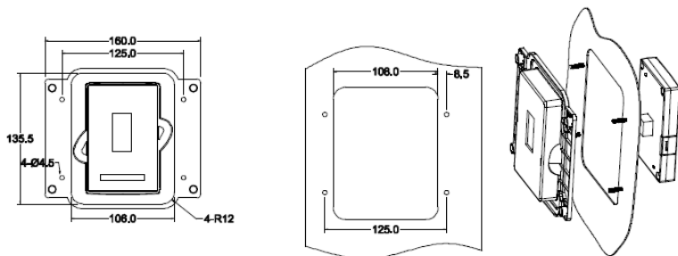
Рисунок В-2 Кронштейн для установки панели управления (стандартная конфигурация) для моделей 037G/045P–500G
