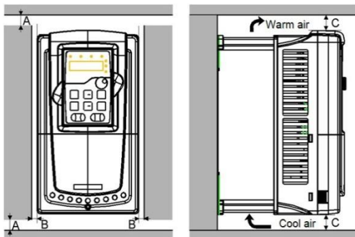
Рис. 4-3 Одиночная установка
