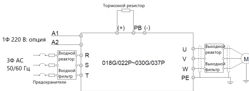
Рис. 4-8 Схема подключения силовых цепей для моделей 018G/022P~030G/037P
