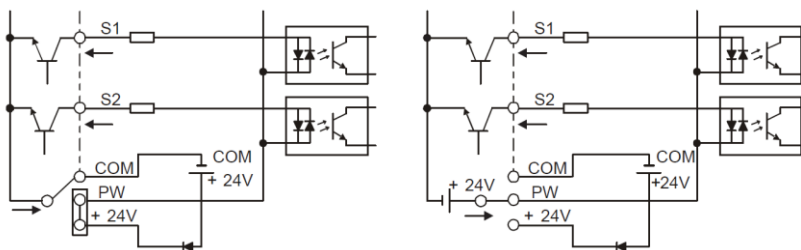
Внутреннее питание (NPN режим)
