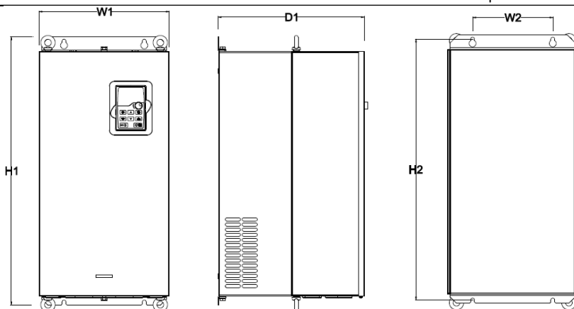
Рисунок В-5 Настенный монтаж для моделей 037G/045P-110G/132P
