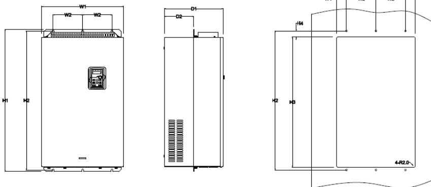
Рисунок В-11 Фланцевый монтаж для моделей 132G/160P-200G/220P
