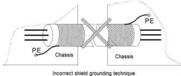
Техника заземления экранированного кабеля
