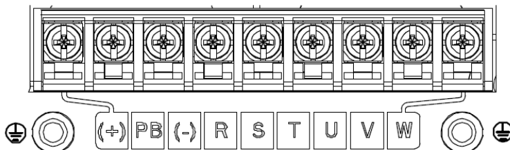
Рис. 4-10 Клеммы силовой цепи для моделей 0R7G-5R5G/7R5P
