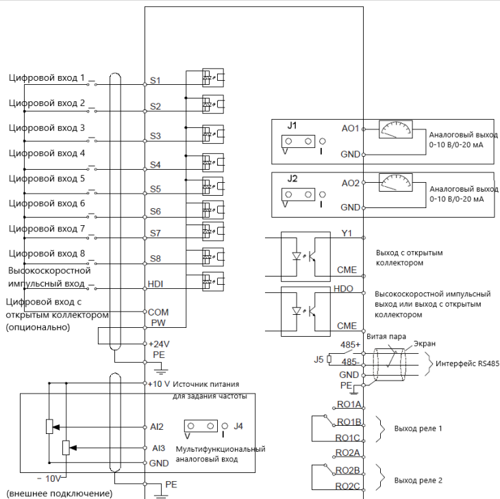
Рис. 4-19. Схема подключения цепей управления и контроля
