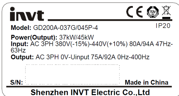
Рис. 3-3 Табличка ПЧ
