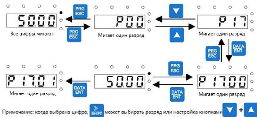
Рис. 5-5 Схема просмотра параметров состояния ПЧ
