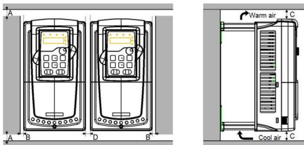
Рис. 4-4 Параллельная установка
