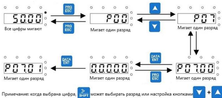
Рис. 5-4 Диаграмма установки пароля
