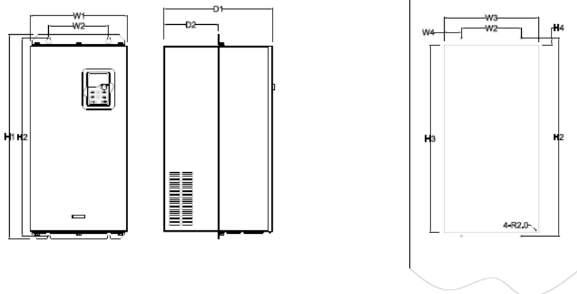
Рисунок В-10 Фланцевый монтаж для моделей 037G/045P-110G/132P
