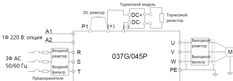
Рис. 4-9 Схема подключения силовых цепей для моделей 037G/045P и выше
