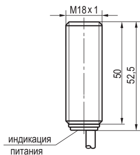
Габаритный чертёж
