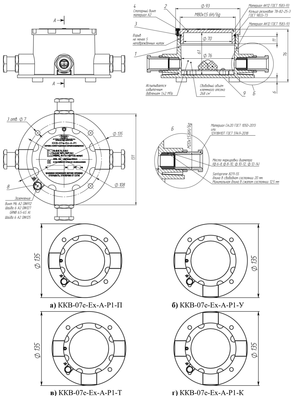
Рисунок 2. Габаритные размеры коробки KKB-07e-Ex-A-P1.
