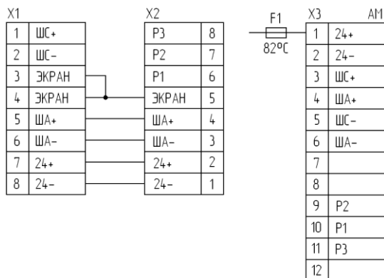
Рисунок 10. Схема соединений клемм на плате ККВ-07е-Ех-А-Р1-БК2 для подключения адресных меток.
