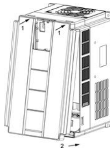
Рис.3-9 Крышка крепления
