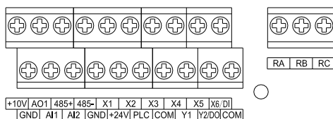
Рис.3-17 Раскладка терминалов управления
