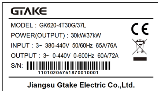
Рис.2-2 Информационная табличка
