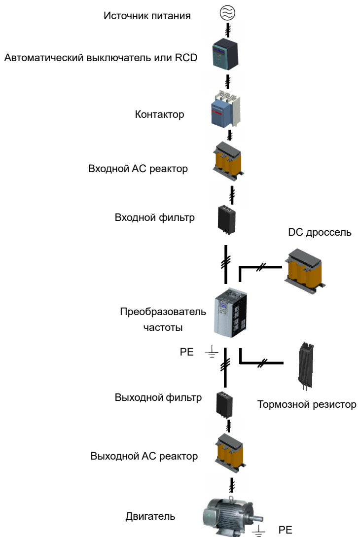
Рис.3-12 Стандартная конфигурация периферийных устройств
