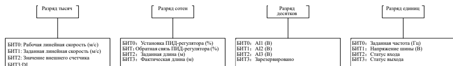
Рис. 4-14. Установка шестнадцатеричного параметра L1-02
