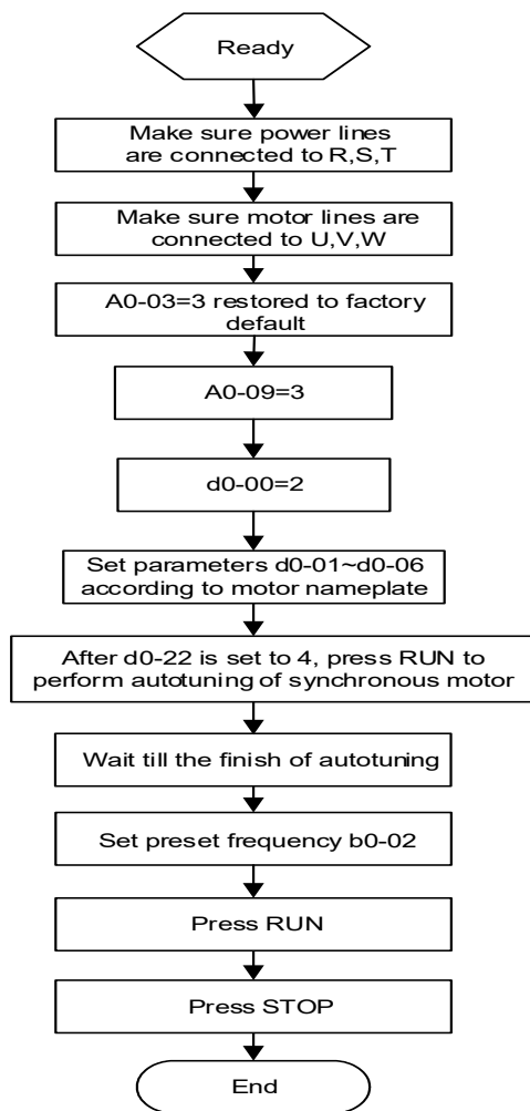
Рис.4-18 Блок-схема первого включения питания для синхронного двигателя
