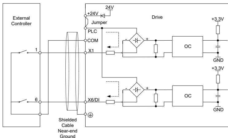
Рис. 3-18 Внутренний источник питания для сухих контактов
