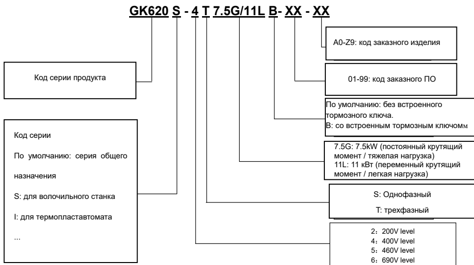
Рис.2-1 Объяснение модели продукта
