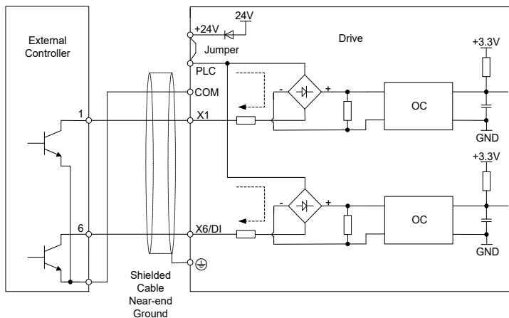
Рис.3-20 Подключение открытого коллектора NPN к внутреннему источнику питания
