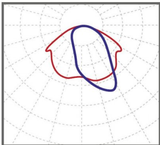
полуширокая Л КСС 130°x45°
