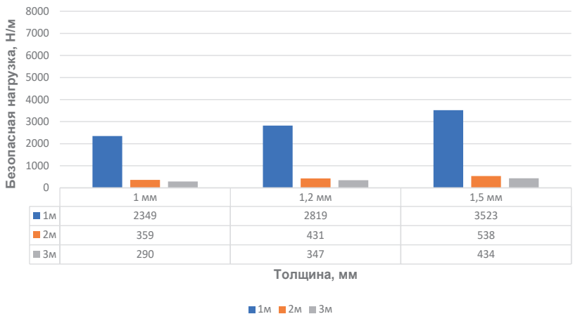
Лоток НЛ-5 борт 24 мм
