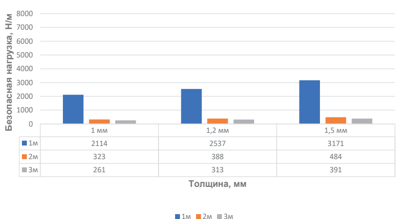
Лоток НЛ 10 борт 24 мм
