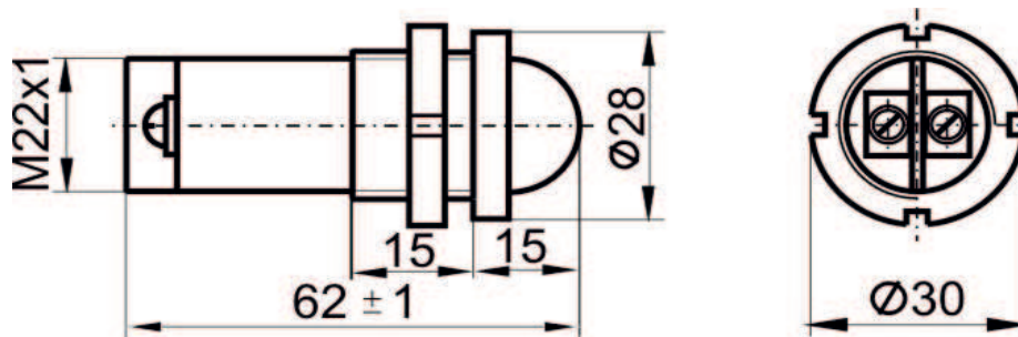
Габаритные размеры
