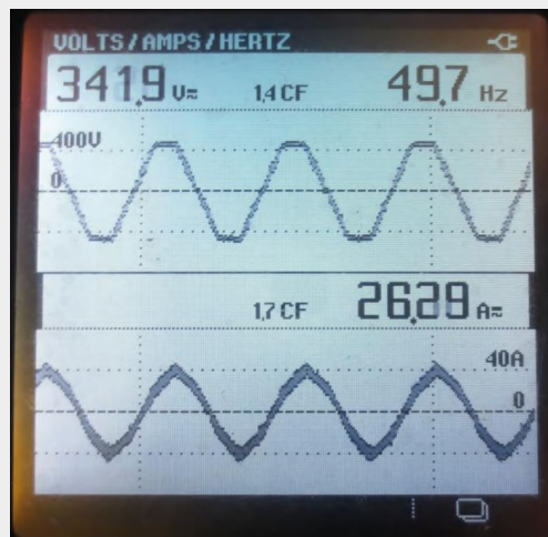
Сигналы тока и напряжения после добавления синус фильтра
