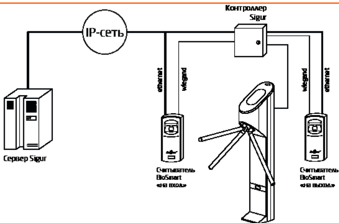
Рис. 335. Пример схемы подключения точки доступа Sigur с биометрическими считывателями BioSmart.
