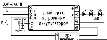
Схема подключения БАП в светильнике ДВО-01-А
