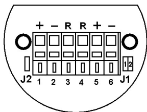
а) ВС-07е-Ех-3(И)-24VDC
