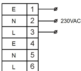
Рисунок 3. Схемы подключения оповещателей BC-07e-Ex-24VDC.
