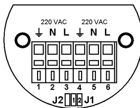
б) ВС-07е-Ех-3(И)-230VAC
