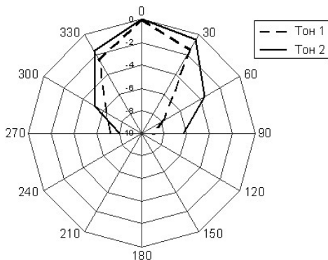
Рисунок 8. Диаграмма направленности звука ВС-07е-Ех-3(И).
