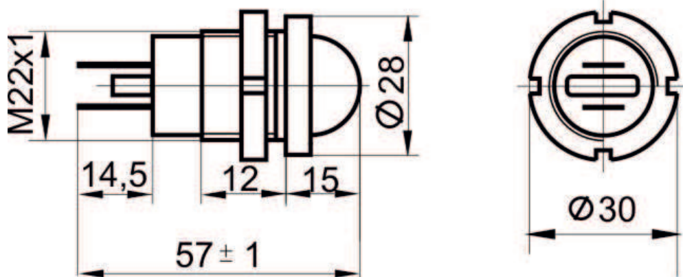
Габаритные размеры
