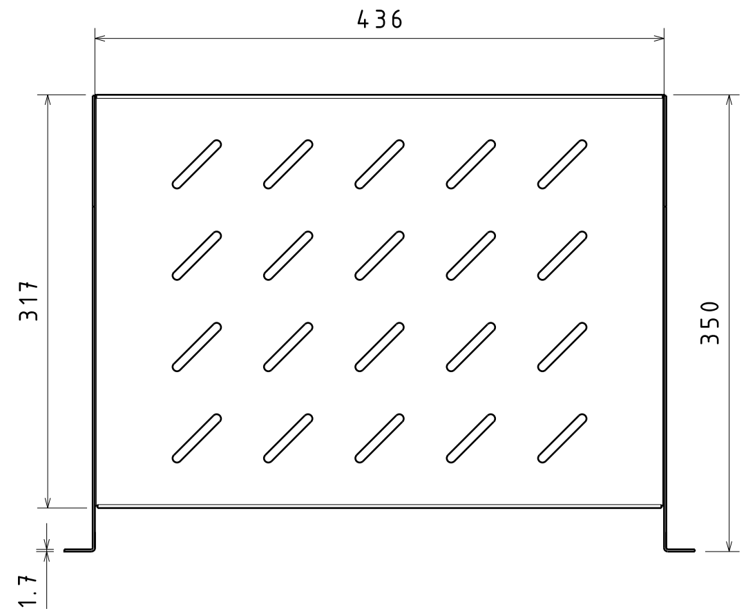
Вид сверху Масштаб: 1:4
