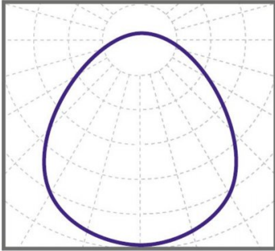
косинусная КСС 90°
