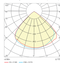
Косинусная КСС (Д90)
