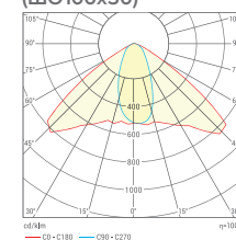
Широкая Осевая КСС (ШО100x50)
