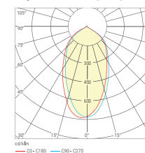
Глубокая КСС (Г60)
