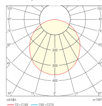
Косинусная КСС (Д120)
