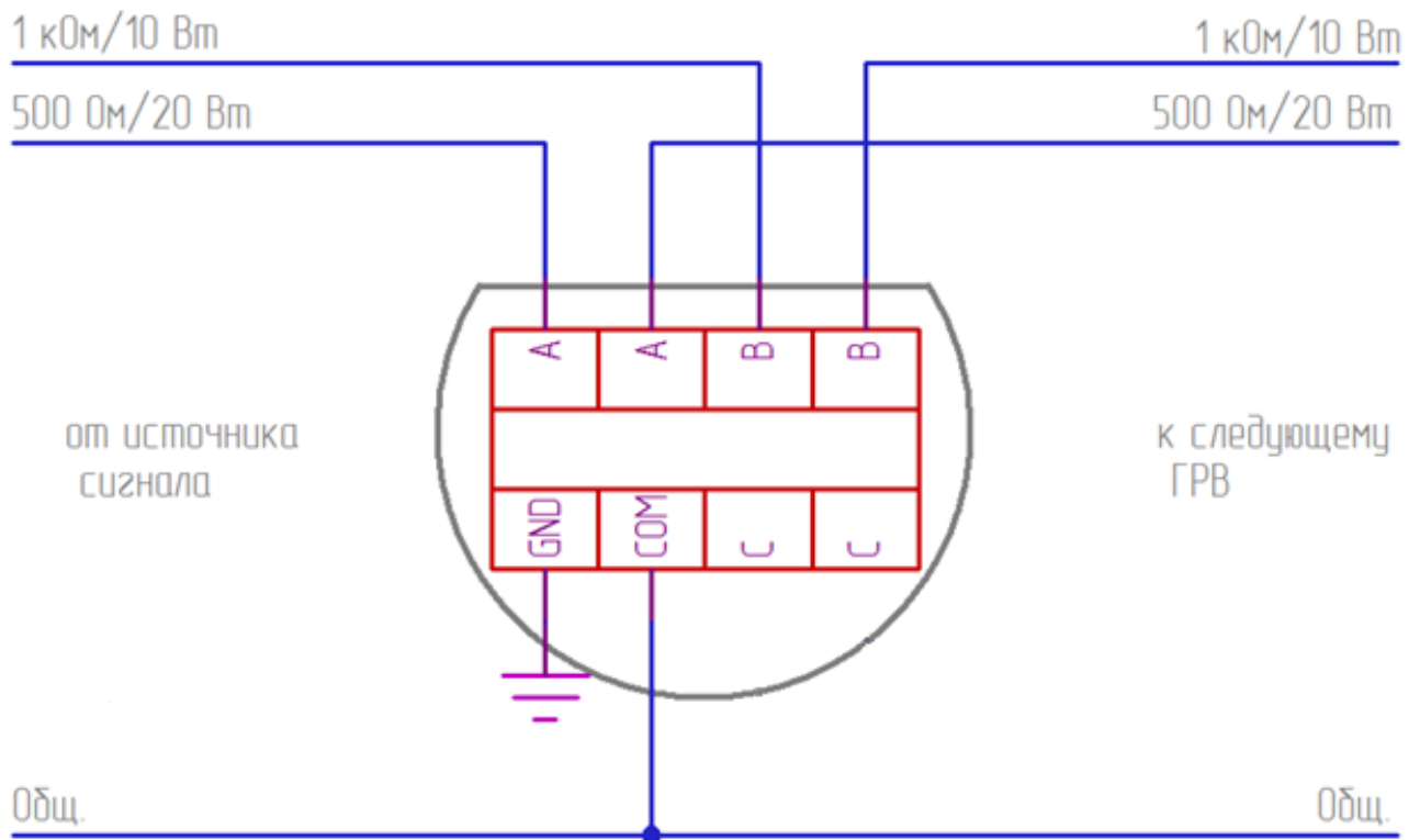
Рисунок Б2 – Схема подключения ГВП-Exd-20
