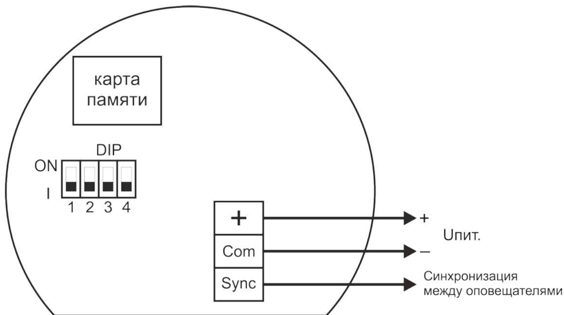
Рис. Б5 – Схема подключения РЗОР-Exd-10, РЗОР-Exd-20, РЗОР-Exd-30, РЗОР-Exd-50
