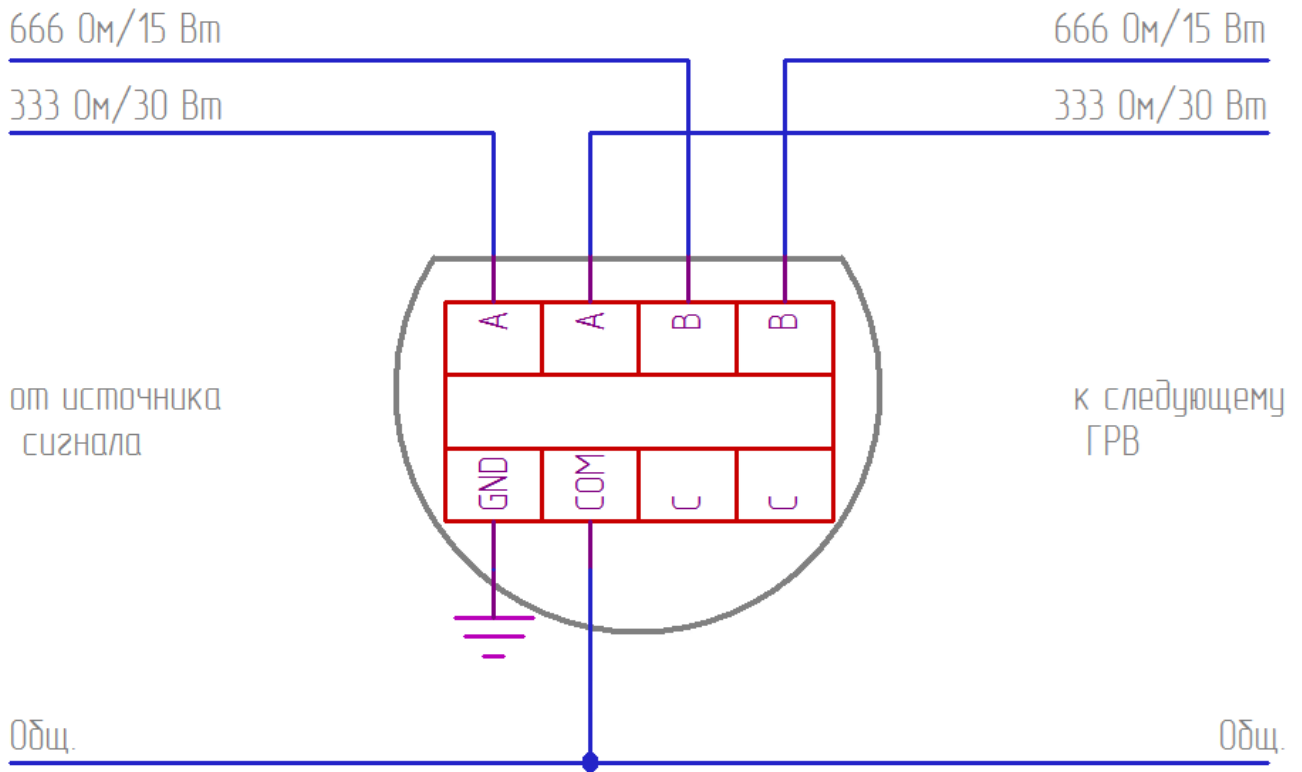
Рисунок Б3 – Схема подключения ГВР-Exd-30
