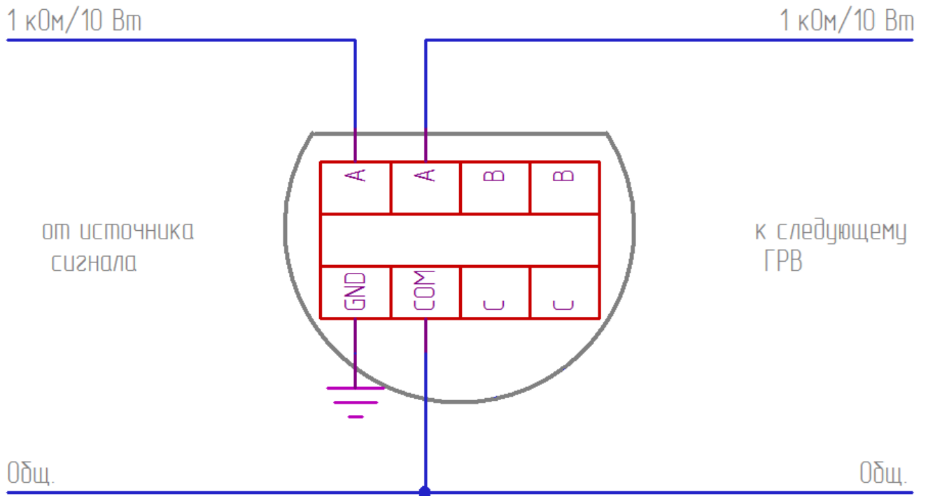
Рисунок Б1 – Схема подключения ГВП-Exd-10
