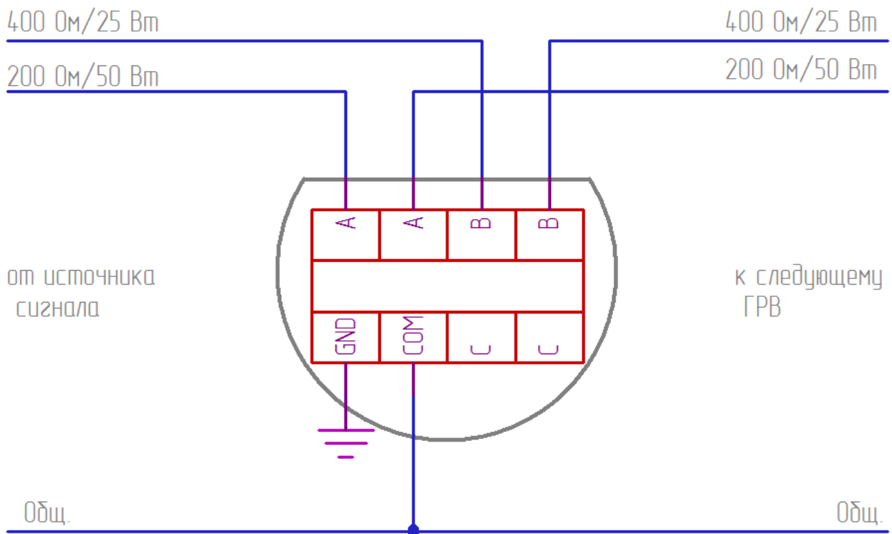
Рисунок Б4 – Схема подключения ГВР-Exd-50
