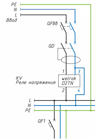
Схема 3. Вариант электрической схемы без транзита нуля через реле welrok D2 TN
