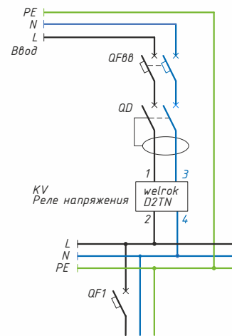
Схема 2. Вариант электрической схемы с транзитом нуля через реле welrok D2 TN
