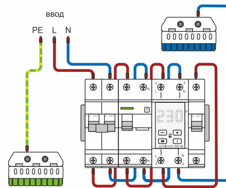
Схема 1. Вариант монтажной схемы с транзитом нуля через реле welrok D2 TN
