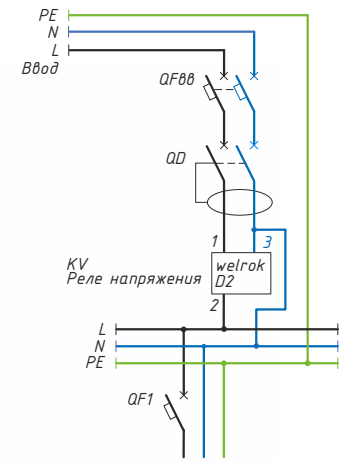
Схема 5. Вариант электрической схемы welrok D2
