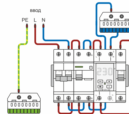
Схема 4. Вариант монтажной схемы welrok D2 и без транзита нуля через реле welrok D2 TN
