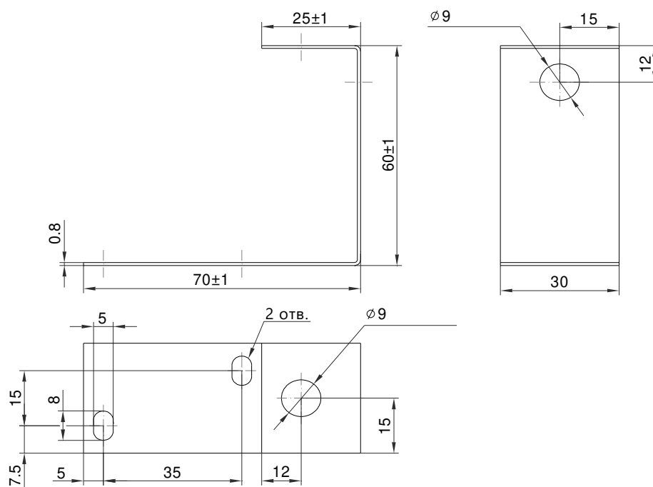
Рисунок 2 - Габаритные и установочные размеры скобы
