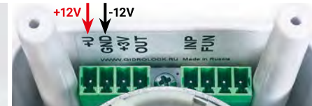
Фото 20. Клеммы разъема электропривода для подключения внешнего блока питания +12 В, проводного выключателя, объединения в систему нескольких шаровых электроприводов
