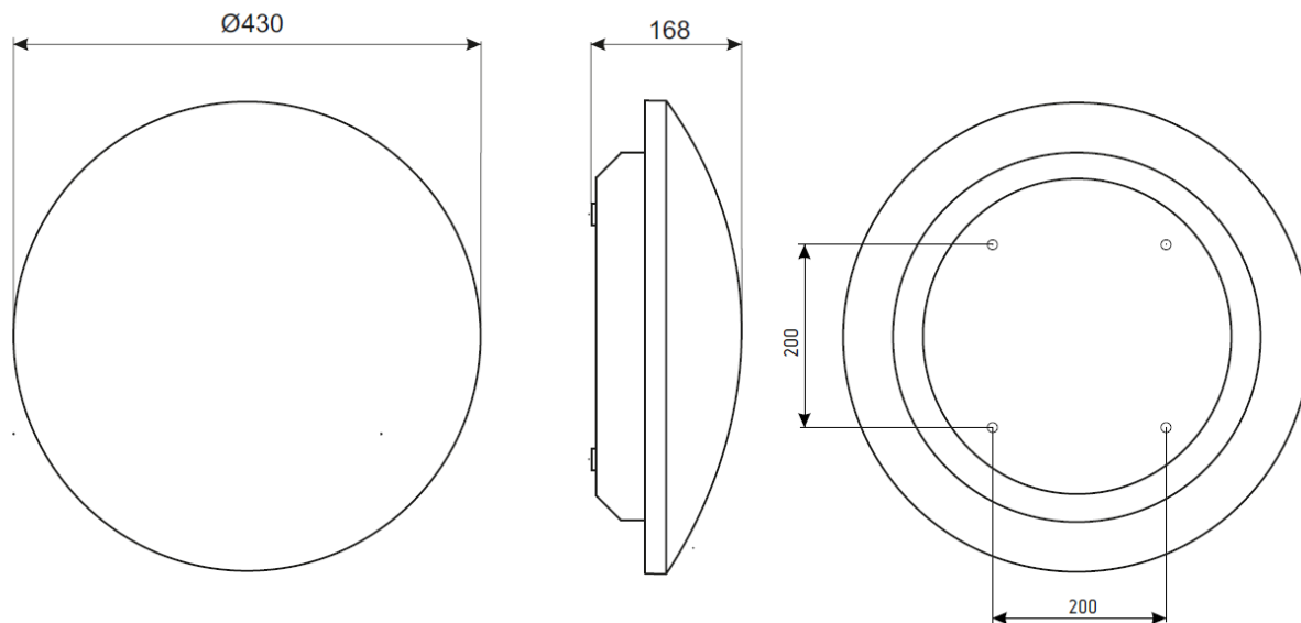
Рис. №2 Габаритный чертёж
