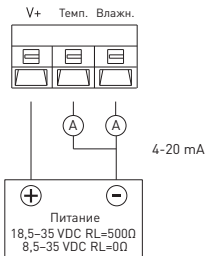
Рис. 12 — Подключение для измерения по току THT-101/102
