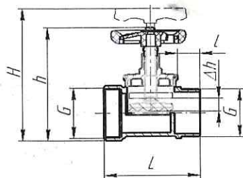
Рисунок 2—Внешний вид прямоточной модели КПЛП, КПЧП и КПКП.
