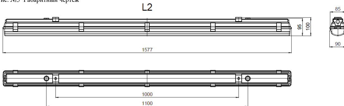
Рис. №5 Габаритный чертёж
