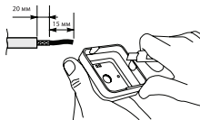
3.3. Зачистить кабель согласно рисунку. Прodelать в крышке отверстие для ввода кабеля согласно его диаметру.
