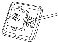
3.4. Отсоединить внутреннюю часть изделия, отжав лезвием отвертки два зажима по бокам механизма.
