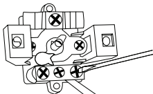
3.5. Присоединить кабель, вставив зачищенные концы в пазы контактных зажимов, затянув винты.
