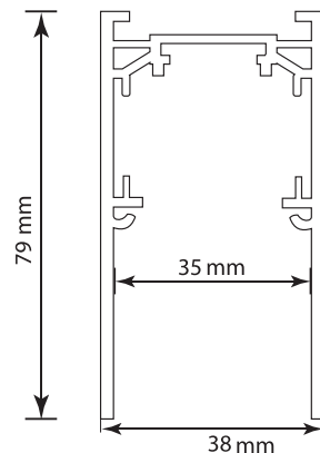
Габариты сечения шинопровода
