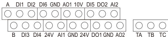
Рисунк 3.10 – Клеммы цепи управления преобразователя
