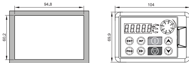
Рисунок 3.15 – Размеры выносной рамки
