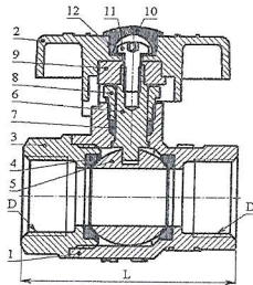
Рисунок 1. Кран КРДШ
