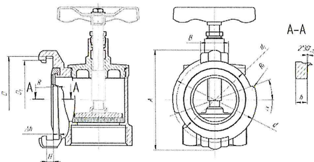
Рисунок 2. Внешний вид соединительной головки клапанов КПАЛ 50, КПАЛ 65.
