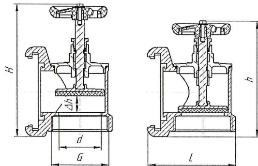
Рисунок 1. Внешний вид клапанов КПАЛ 50, КПАЛ 65
