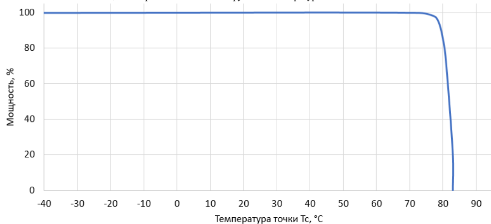
Зависимость мощности при максимальной нагрузке от температуры точки Tc.
