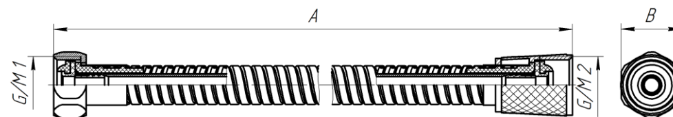
Рисунок 1 – Габаритные и присоединительные размеры изделия
