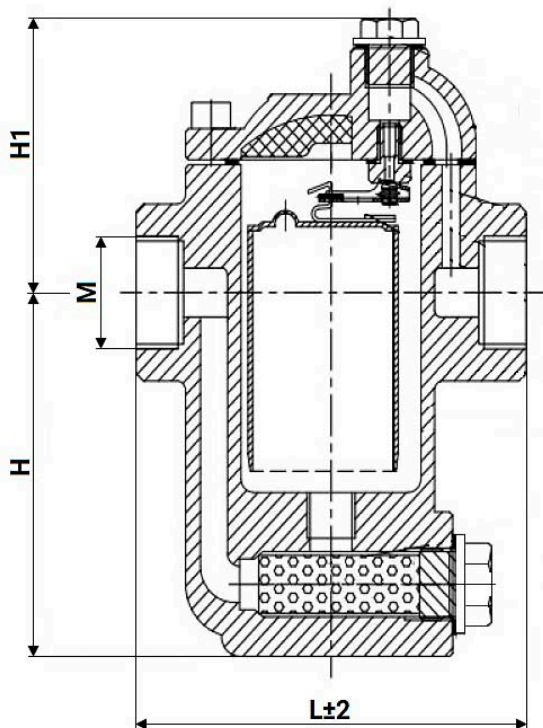
Рисунок 2 – Размеры
