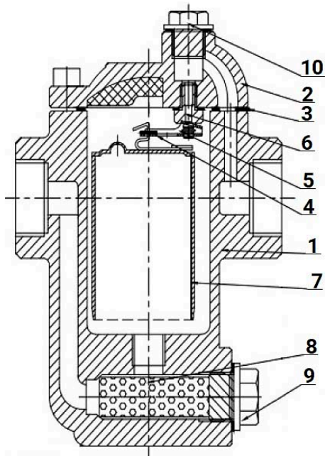
Рисунок 1 – Деталировка
