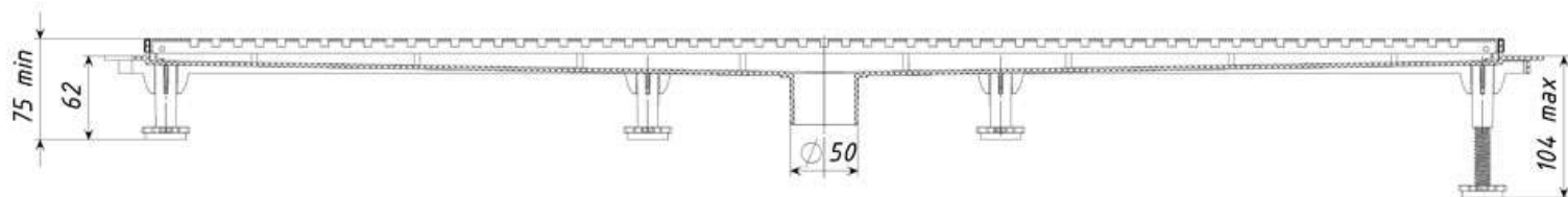
Вариант установки без затвора
