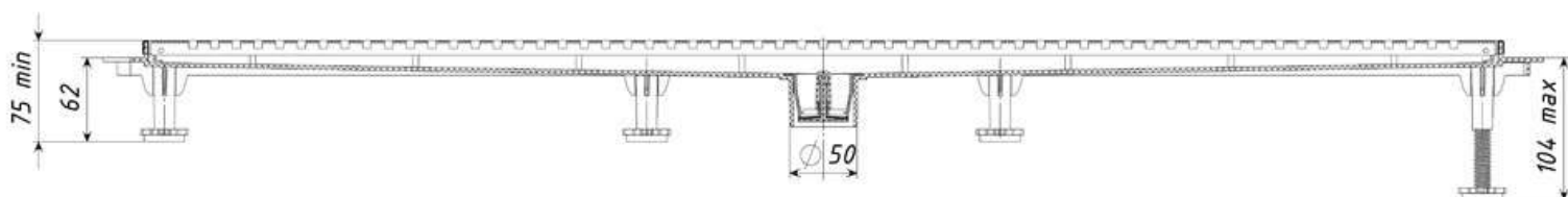
Вариант установки механического "сухого" затвора
